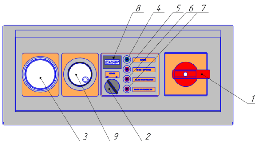
Рис. 3. Панель управления
