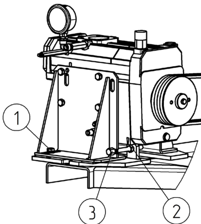
Рис.4.5 Натяжение ремней
