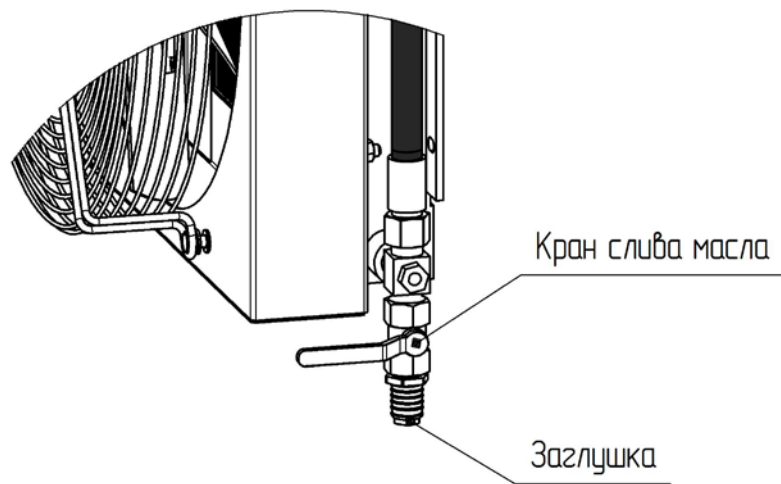
Рис. 6. Маслоохладитель
