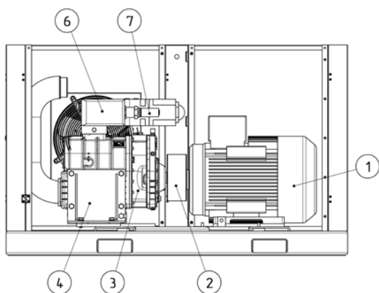
Рис. 2. Общий вид установки
